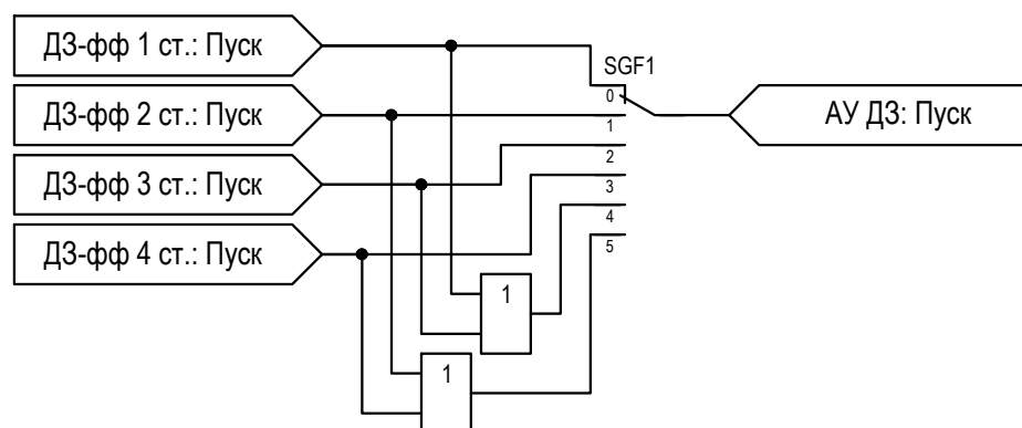
Рисунок 2.9 – Функциональная схема логики АУ Д3
